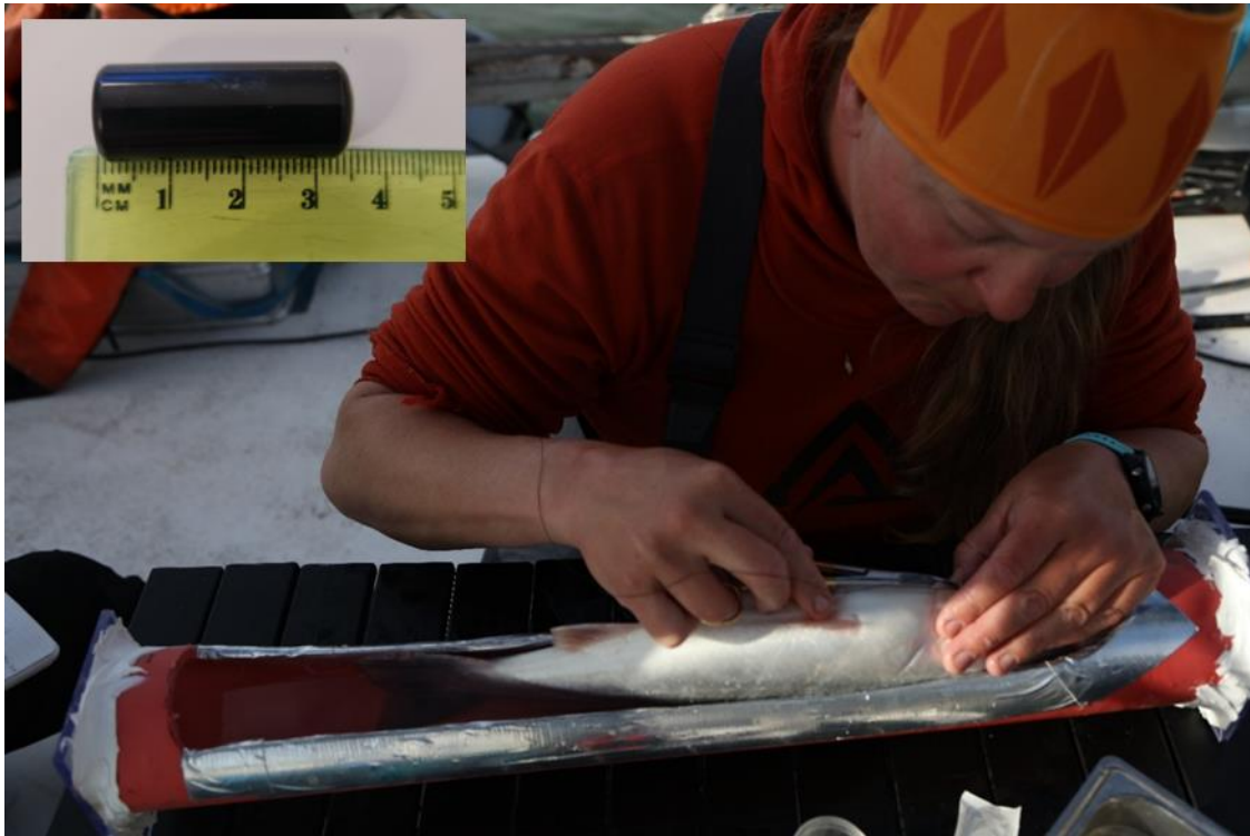
Figur 3. Merking av sjørøye. Bilde oppe til venstre viser et akustisk MP-13 merke med en lengde på 33 mm. Foto: Akvaplan-niva.
